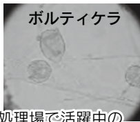
下水処理場で活躍中の 微生物の例
