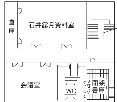
2階平面図
