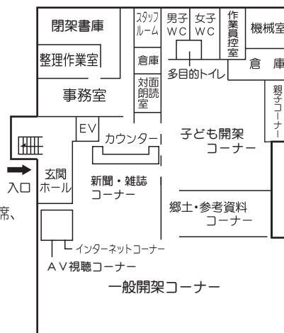
1階平面図
