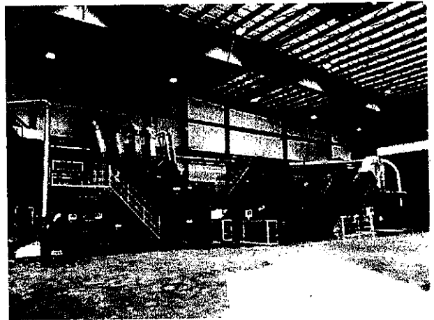
集められたペットボトルを破砕する工程の機械
