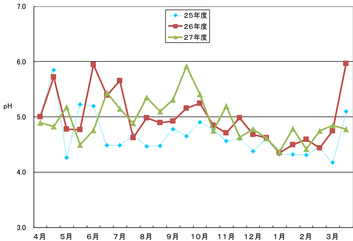
図 1－37 酸性雨・酸性雪のpH（月平均値）の変化（4～12月は山王、1～3月は八橋で調査）
