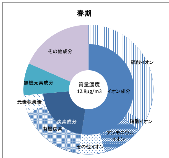
図1-28 PM2.5成分分析結果(春期) (平成27年度)
