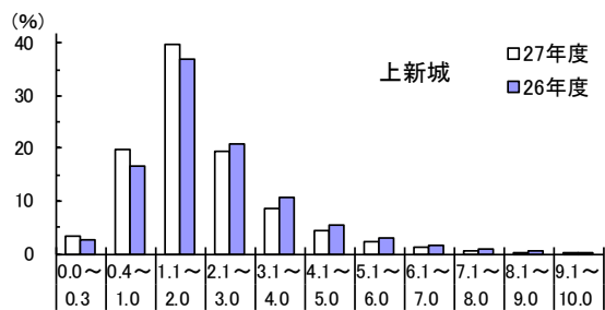
図 1 - 5 風速別出現図
