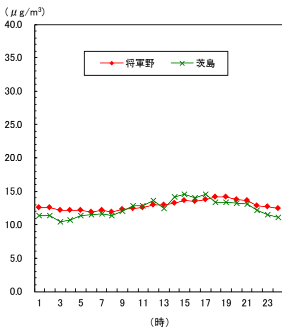
図1-27 微小粒子状物質の時刻平均値の変化 (平成27年度)
