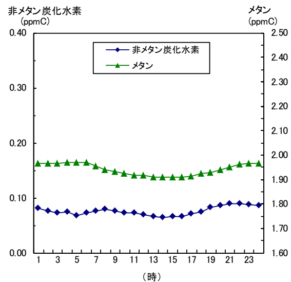
図 1-33 非メタン炭化水素とメタンの時刻平均値の変化（平成 27 年度）
