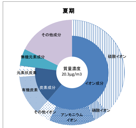
図1-29 PM2.5成分分析結果(夏期) (平成27年度)
