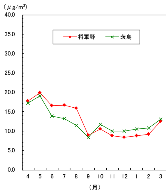
図1-26 微小粒子状物質の月平均値の変化 (平成27年度)
