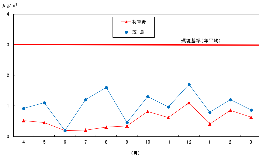
図1-36 ベンゼンの測定結果(平成27年度)
