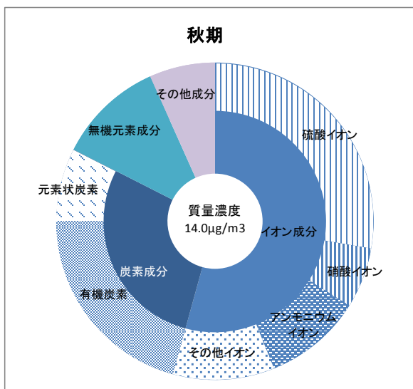
図1-30 PM2.5成分分析結果(秋期) (平成27年度)
