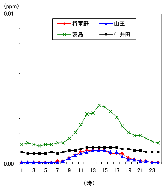
図1-9 二酸化硫黄時刻平均値の変化(平成27年度)
