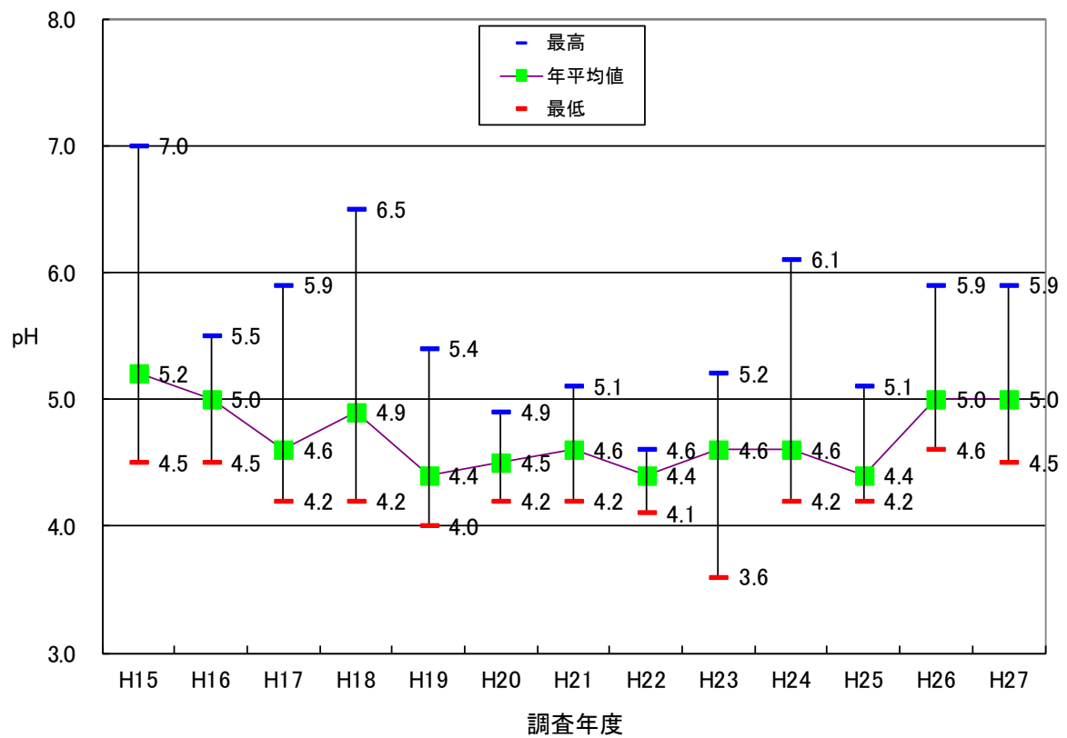
図 1－38 酸性雨（山王）の平均値経年変化
