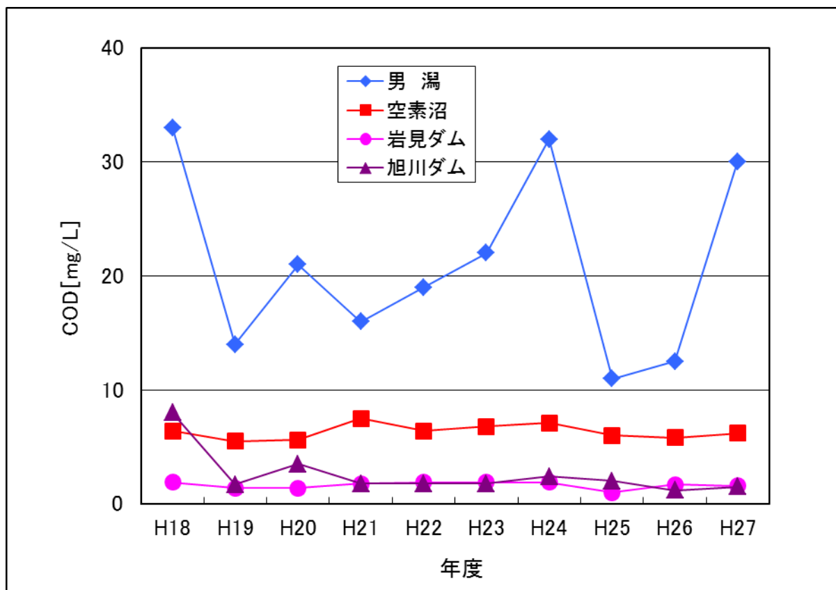
図 2-5 湖沼のCOD75%値の経年変化
