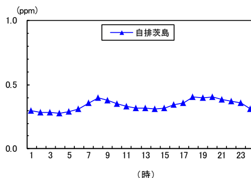
図 1－21 一酸化炭素の時刻平均値の変化 （平成 27 年度）
