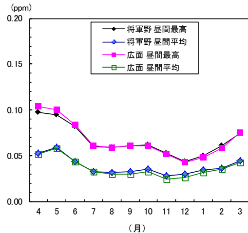
図1-23 光化学オキシダントの月平均値の変化（平成27年度）
