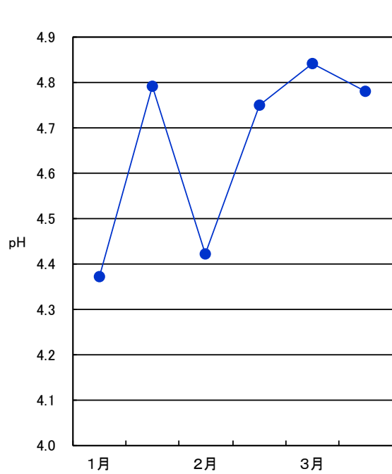
図 1-40 降雪のpHの推移
