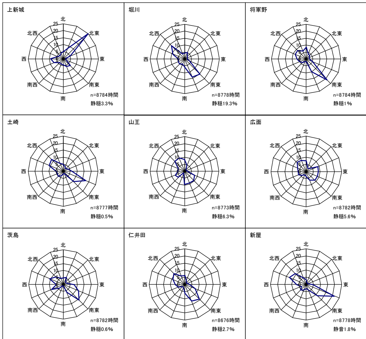
図1－4 風配図（平成27年度）
