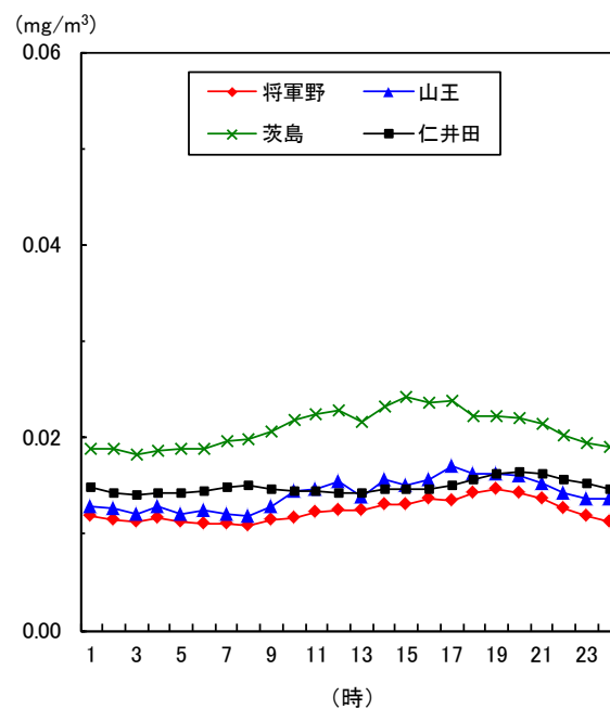
図1-18 浮遊粒子状物質の時刻平均値の変化 (平成27年度)
