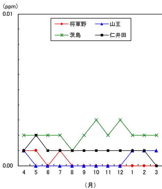
図1-8 二酸化硫黄月平均値の変化(平成27年度)
