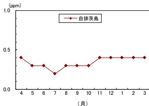
図 1－20 一酸化炭素の月平均値の変化 （平成 27 年度）
