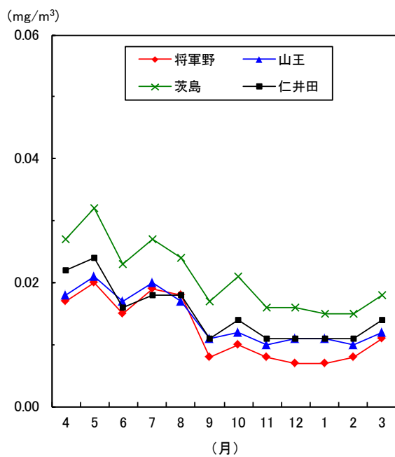
図1-17 浮遊粒子状物質の月平均値の変化 (平成27年度)
