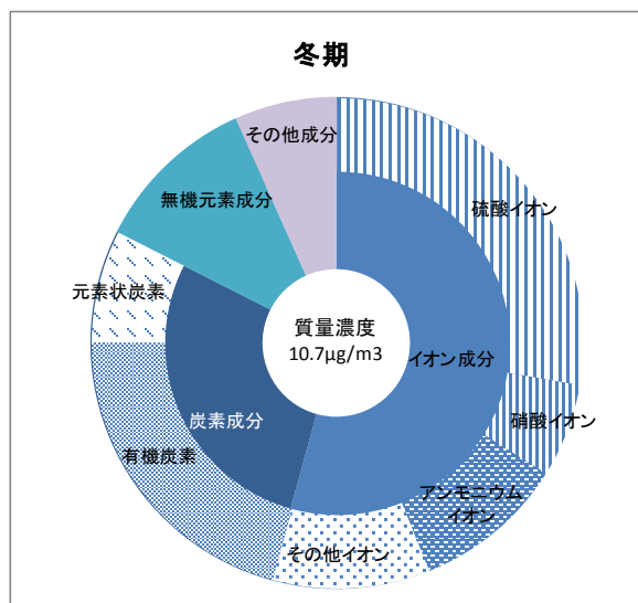
図1-31 PM2.5成分分析結果(冬期) (平成27年度)
