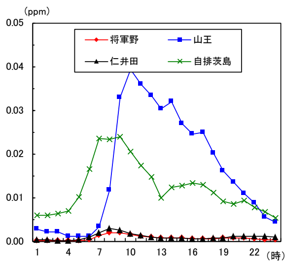
図1-12 一酸化窒素時刻平均値の変化 (平成27年度)
