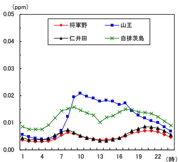
図1-13 二酸化窒素時刻平均値の変化 (平成27年度)
