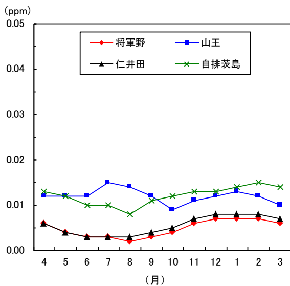
図1-14 二酸化窒素月平均値の変化 (平成27年度)
