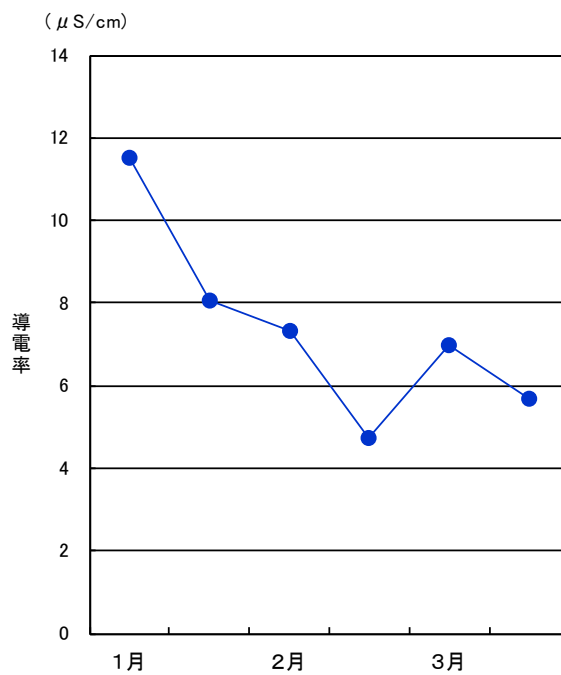
図 1-41 降雪の導電率の推移
