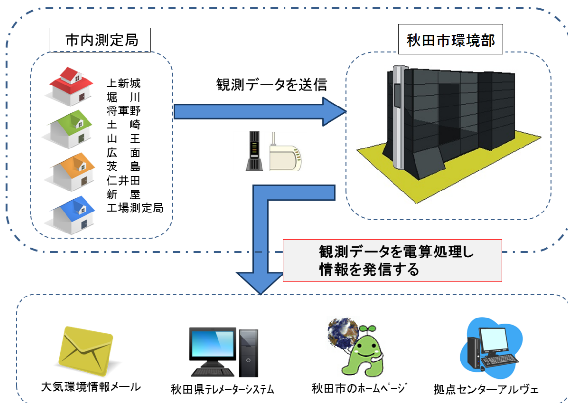
図 1-2 テレメーターシステムの概要
