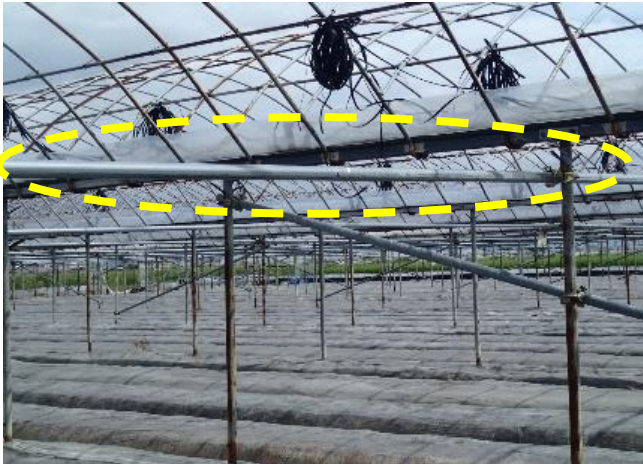
タイバーの設置による補強
