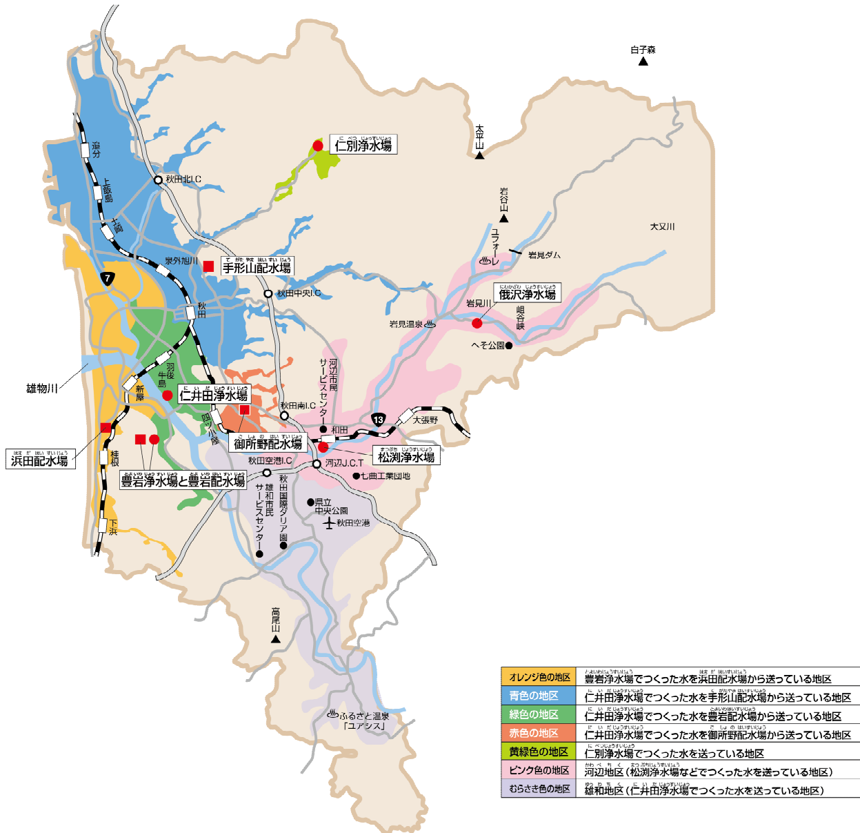
資料 28-1 給水区域および主要施設配置図
