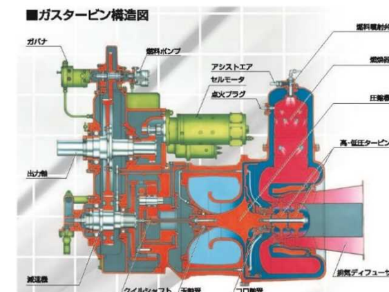
【ガスタービン構造図】
