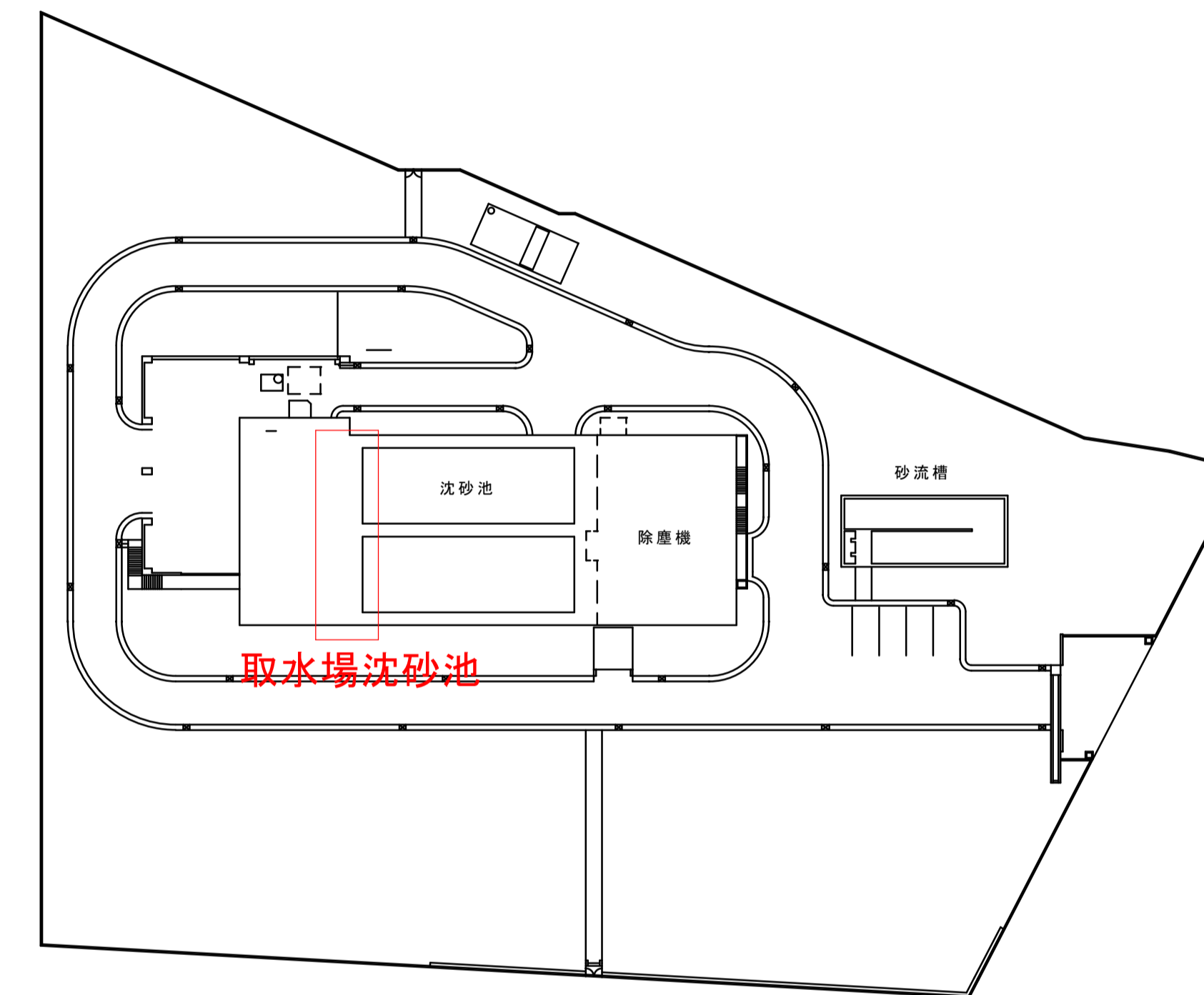
豊岩取水場全体平面図 S=1/500
