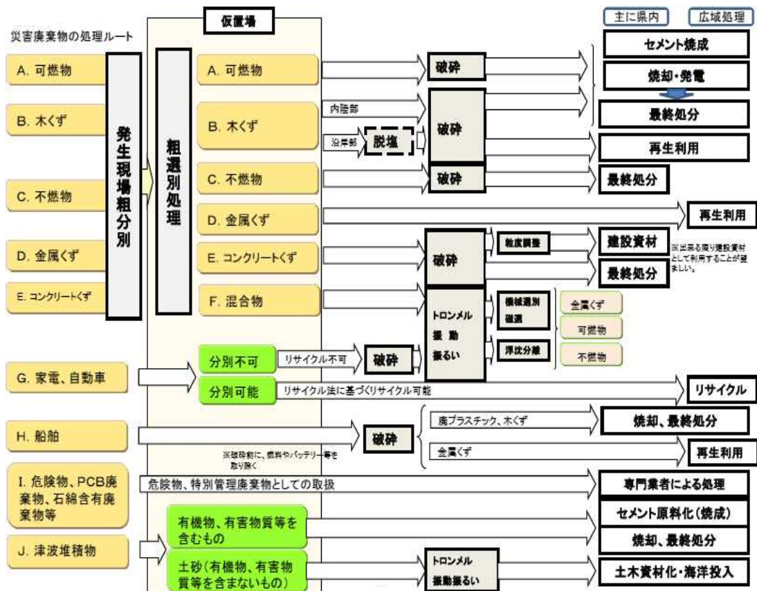
図 3-13-1 災害廃棄物処理フロー図
