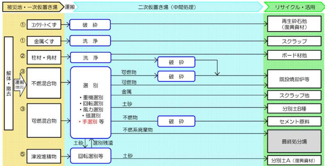
図 3-14-2 二次仮置き場における標準的な中間処理フロー（岩手県）抜粋
