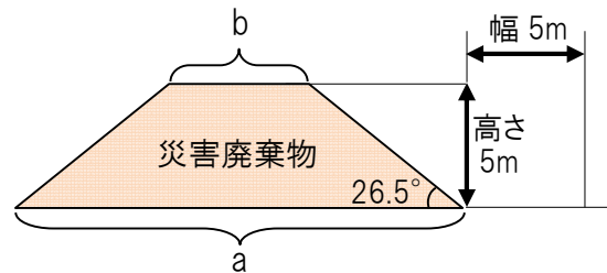
横断面図
