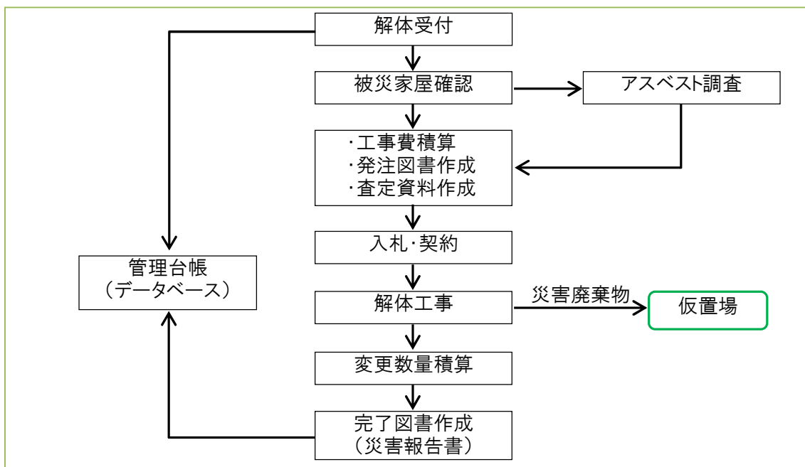
図 3-15-1 緊急解体以降の被災家屋等の解体・撤去の流れ
