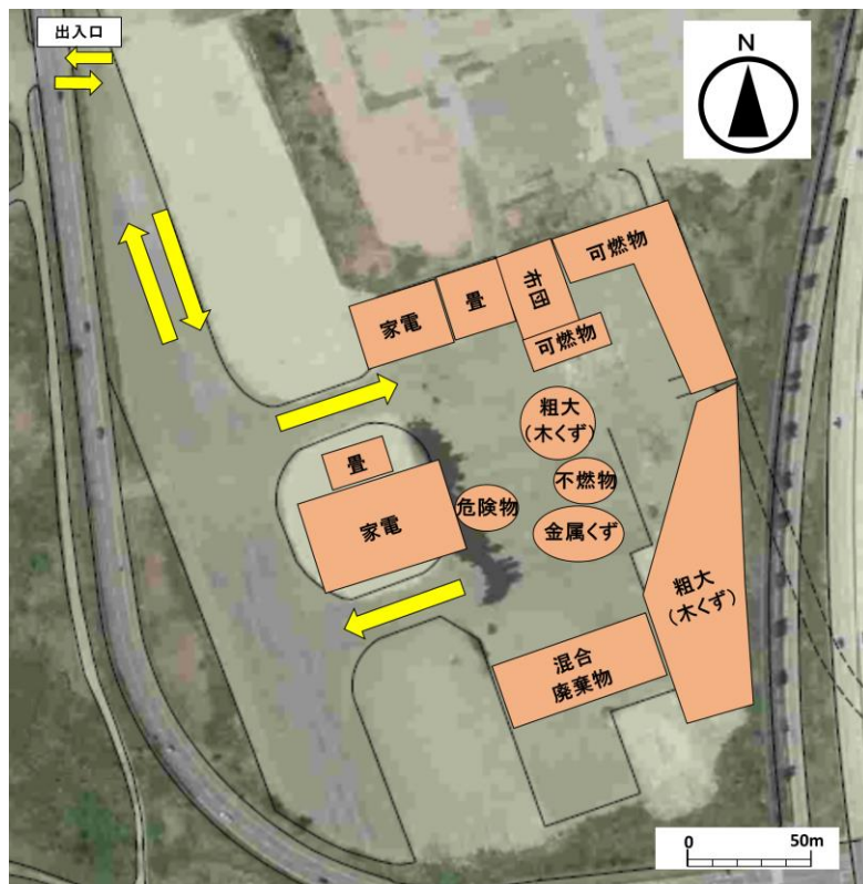
図 2-6-1 一次仮置場のレイアウト例（令和 5 年 7 月 豪雨 秋田市 旧空港跡地）
