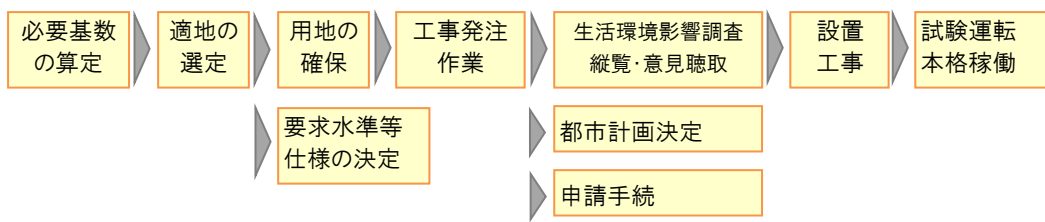
仮設焼却施設等の設置フロー (例) 出典：「災害廃棄物対策指針(環境省 平成30年3月) 修正
