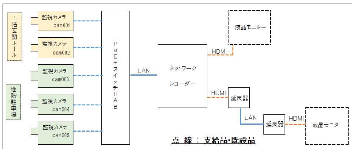
ブロック図
