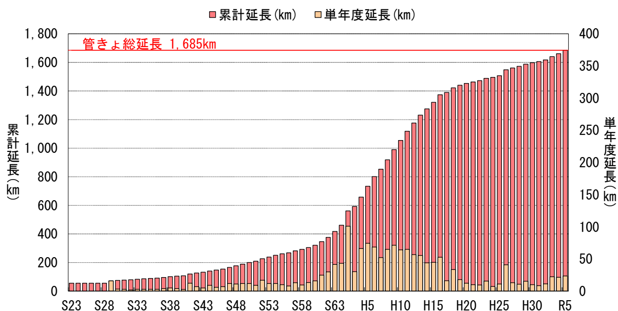
図表３－９ 年度別管きょ延長の推移（公共下水道）
