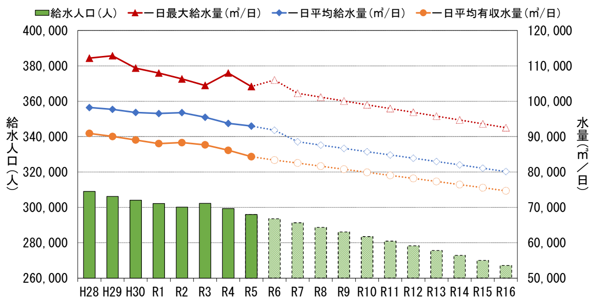
図表４－４ 給水人口と給水量の実績と予測
