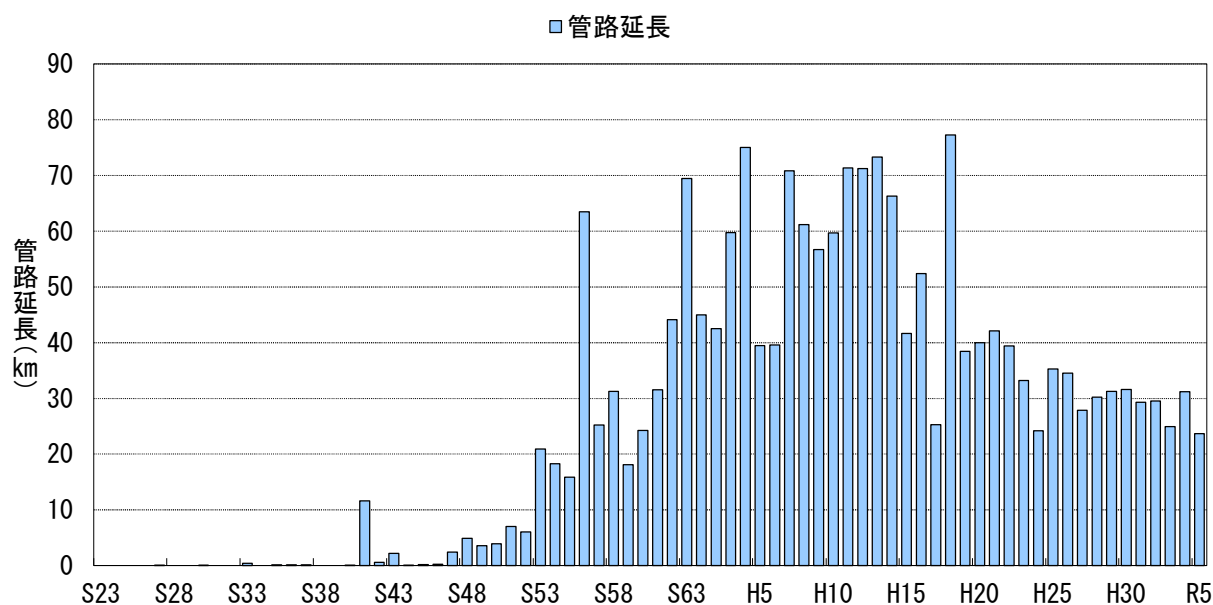
図表３－５ 年度別管路延長の推移
