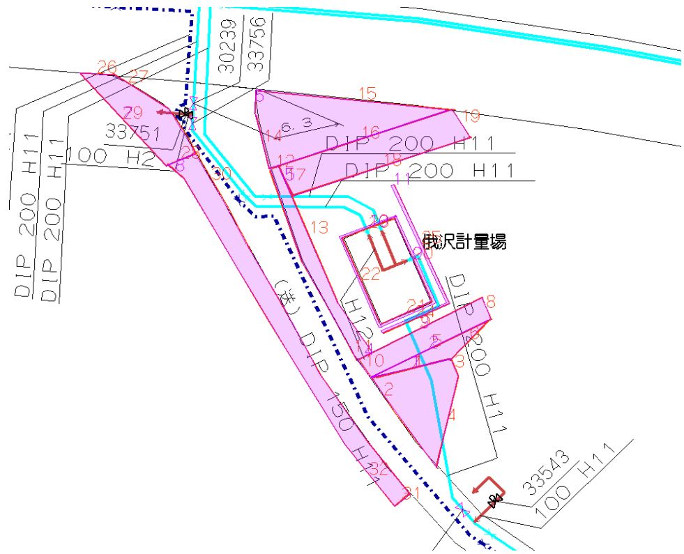
平面図
