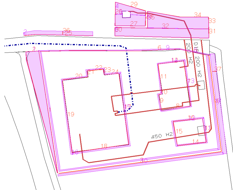
平面図
