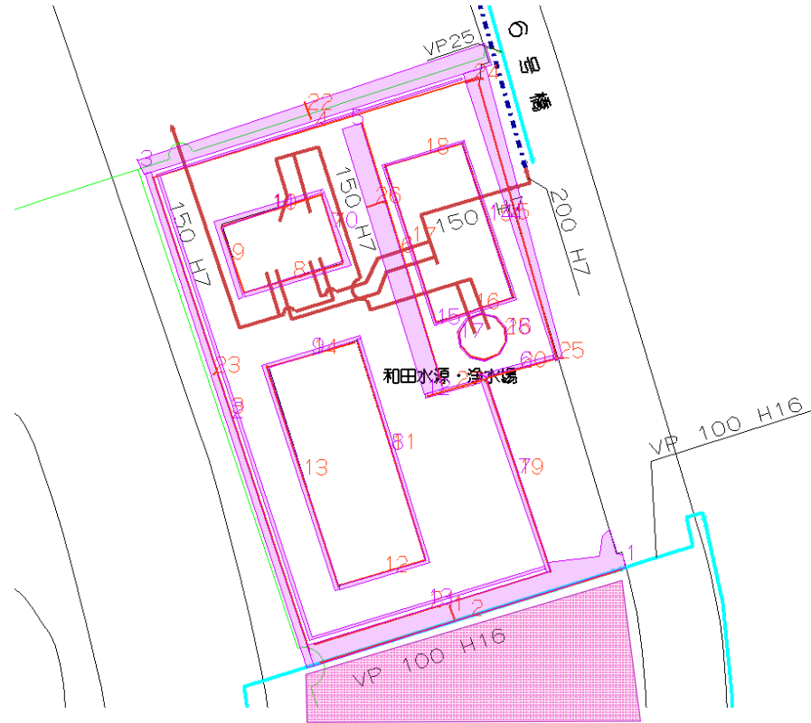
平面図
