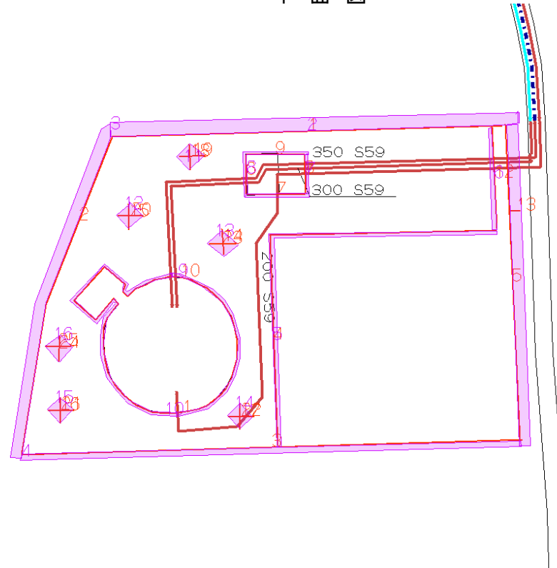
平面図
